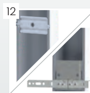
Elementy wzmacniające konstrukcję ościeżnicy z kotwami montażowymi lub bez 12. Ościeżnica 10/54,11/54 13. Ościeżnica 15/54
