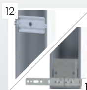
Elementy wzmocniające konstrukcję ościeznicy z kotwami montażowymi lub bez 12. Ościeznica 10/54/11/54 13. Ościeznica 15/54
