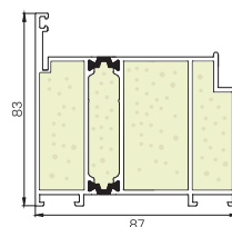
PROFIL OŚCIEŻNICY
