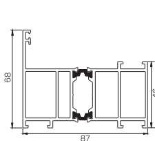
PROFIL NAŚWIEITŁA
