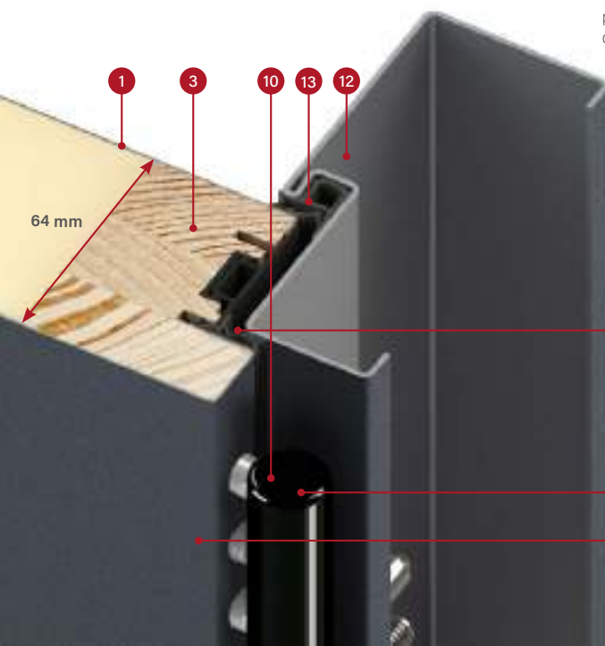
przekrój ościeżnicy stalowej dla skrzydła THERMO 64
