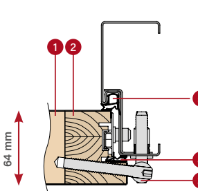
OŚCIEŻNICA STALOWA
