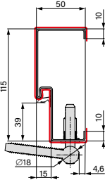
OŚCIEŻNICA STALOWA
