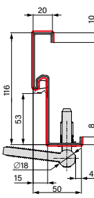
OŚCIEŻNICA STALOWA NAROŻNA
