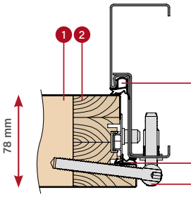
OŚCIEŻNICA STALOWA
