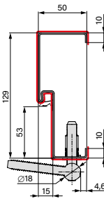
OŚCIEŻNICA STALOWA
